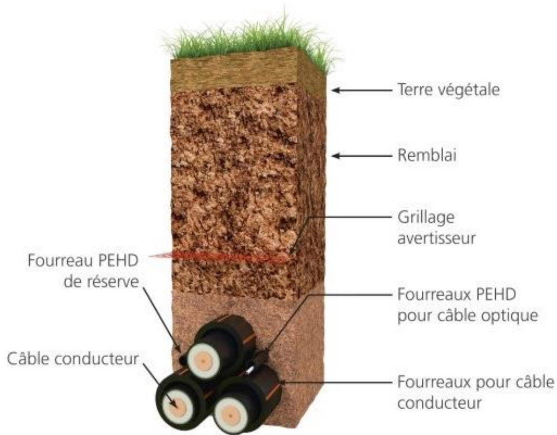
Schéma de pose en fourreaux PEHD
